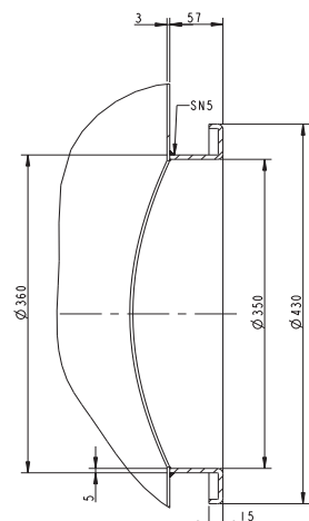
PARTICOLARE ATTACCO FLANGIATO (Scala 1:5)
