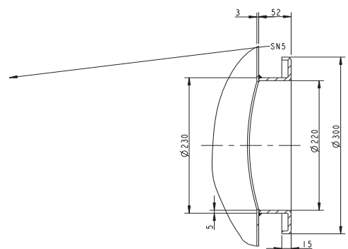
PARTICOLARE ATTACCO FLANGIATO (Scala 1:5)
