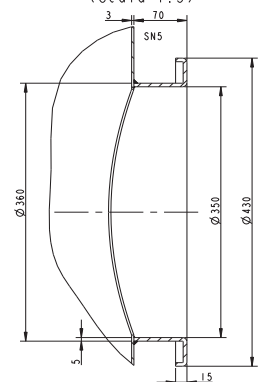
PARTICOLARE ATTACCO FLANGIATO (Scala 1:5)
