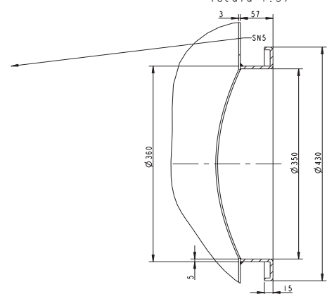
PARTICOLARE ATTACCO FLANGIATO (Scala 1:5)
